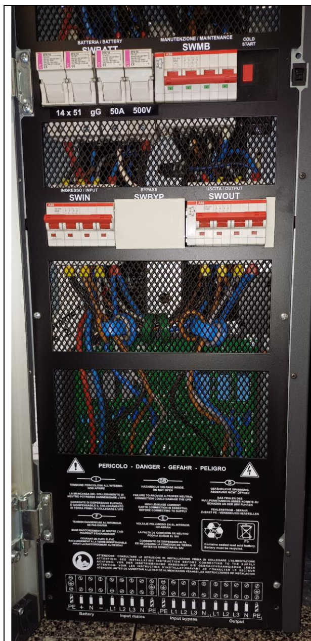
Figura 1 - Fronte interna dopo apertura dello sportellino dei tre UPS sala server
