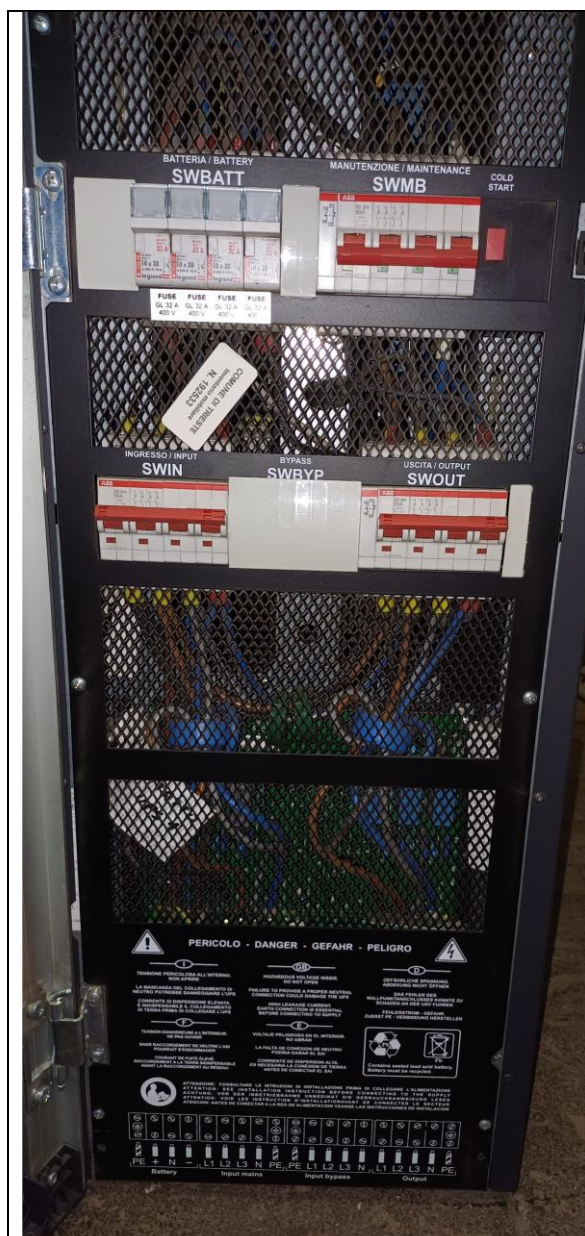
Figura 2 - Fronte interna dopo apertura dello sportellino dei due UPS sala server centrale telefonica
