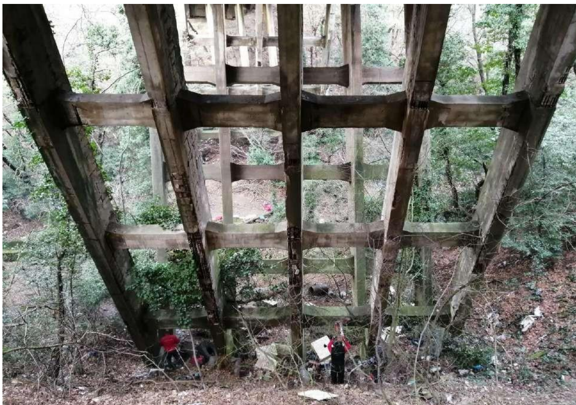
Corrosione dei ferri d'armatura ed espulsione del copriferro dei pilastri.
