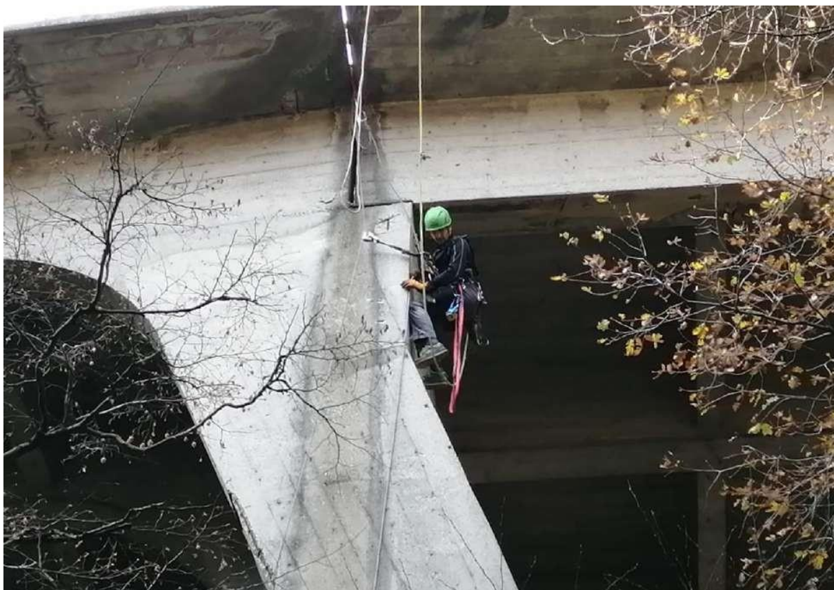
Infiltrazione di acqua piovana sui pilastri.
