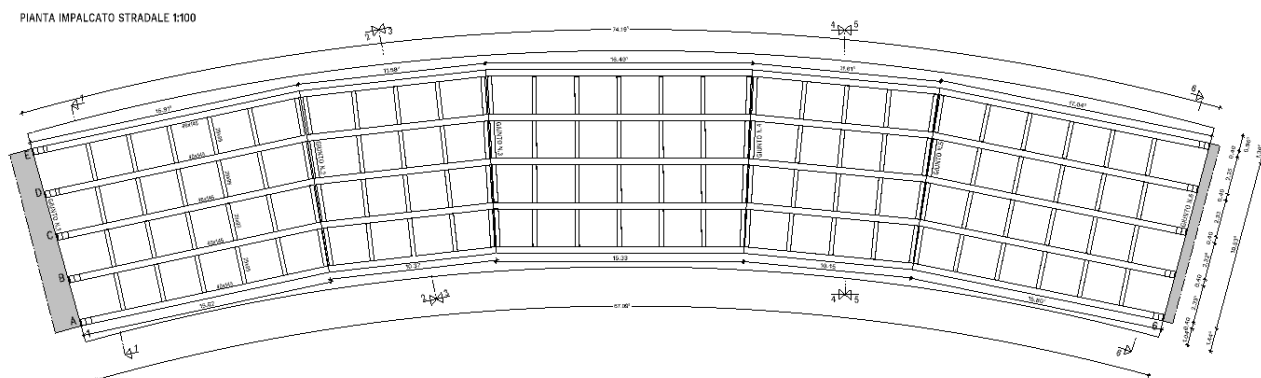
Pianta del ponte con graticcio di travi.
